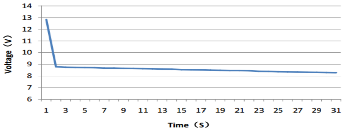
Cold Cranking Test Graph (-18°C, 500CCA)
