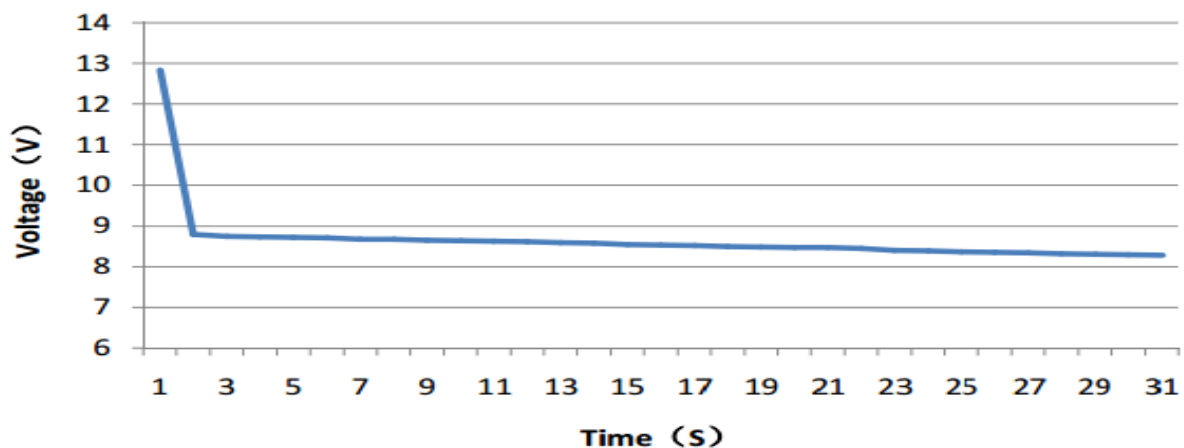
Cold Cranking Test Graph (-18°C, 500CCA)
