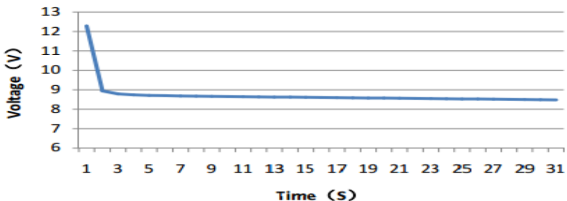
Cold Cranking Test Graph (-18°C, 712CCA)
