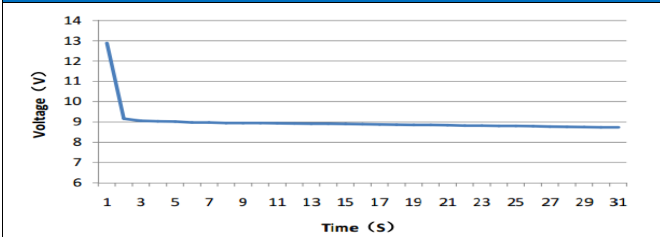
Cold Cranking Test Graph (-18°C, 1000CCA)
