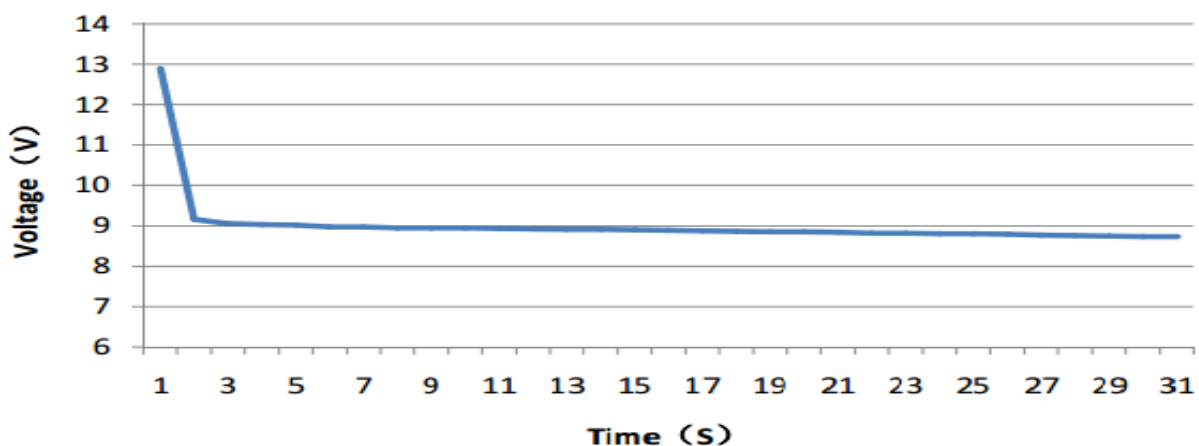
Cold Cranking Test Graph (-18°C, 1100CCA)
