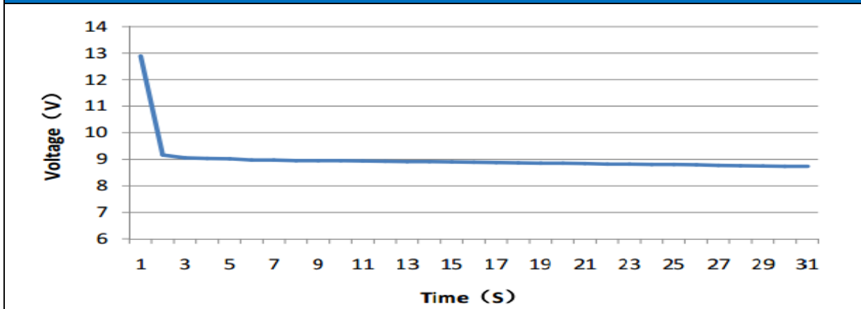
Cold Cranking Test Graph (-18°C, 900CCA)
