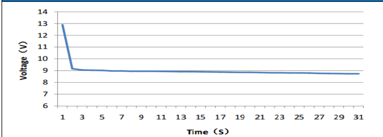
Cold Cranking Test Graph (-18°C, 1000CCA)
