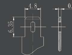
F1 Terminal
